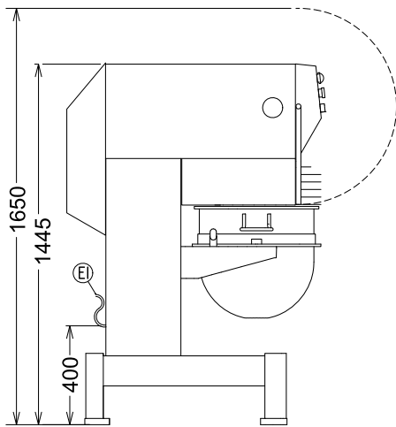
Oldalnézet
